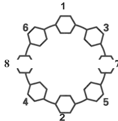
8-Lug Bolt Pattern
